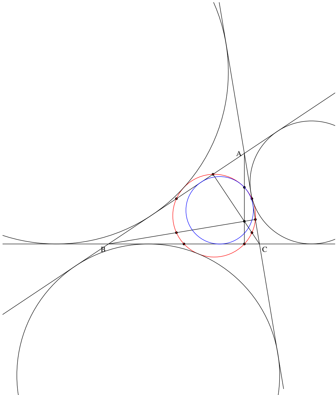
図 1 九点円, 内接円, 傍接円
